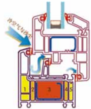
北新暖静门窗五腔室三密封结构图
